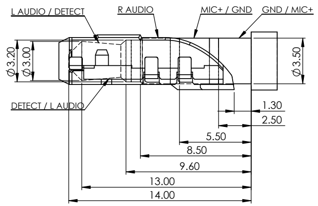
PLUG插入示意图
